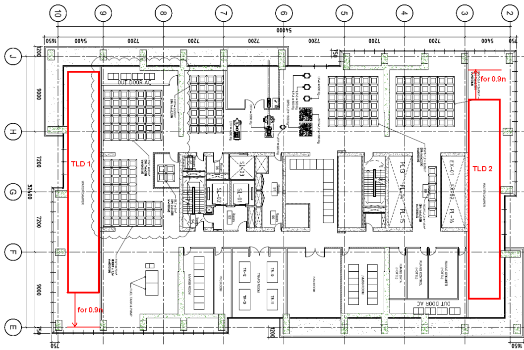
(a) Layout in Plan (Level 44) 分布图 (44层)
